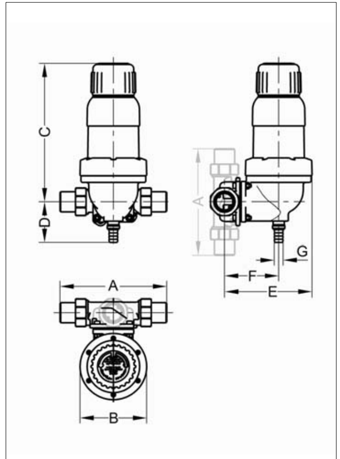
Abb. 9: Einbaumaße JPF + 1 1/2" - 2"
