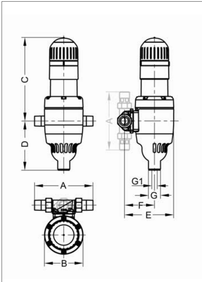
Abb. 8: Einbaumaße JPF + 3/4" - 1 1/4"
